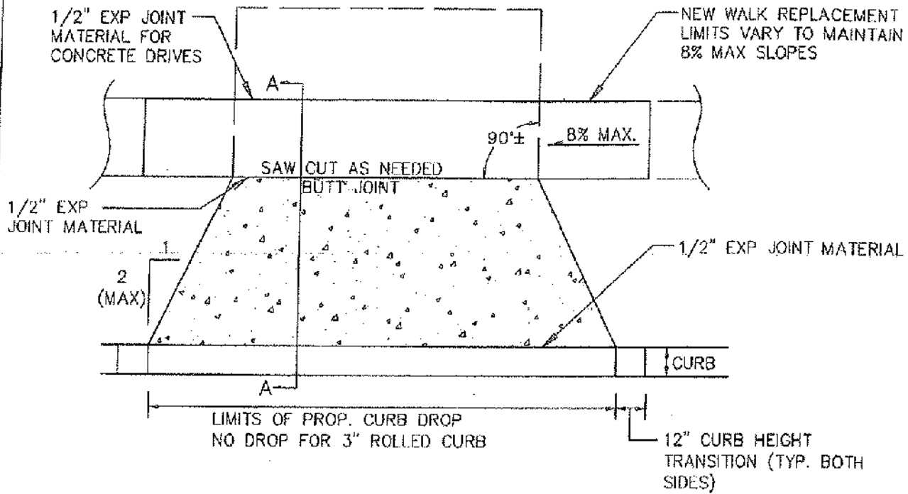
DRIVEWAY APRON N.T.S.
