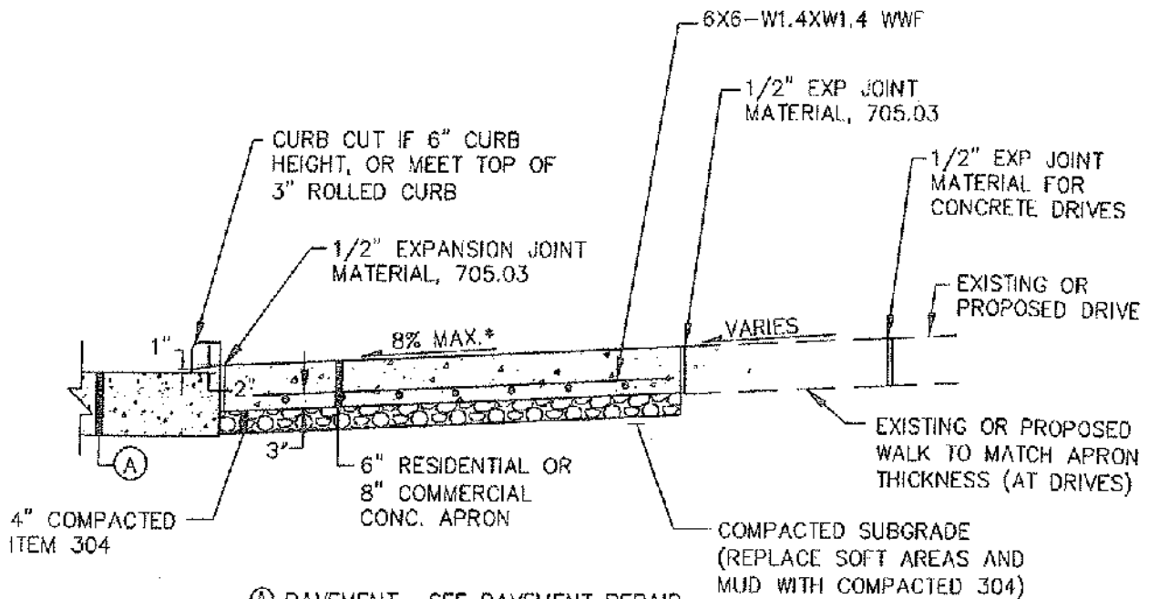
DRIVEWAY APRON N.T.S.
