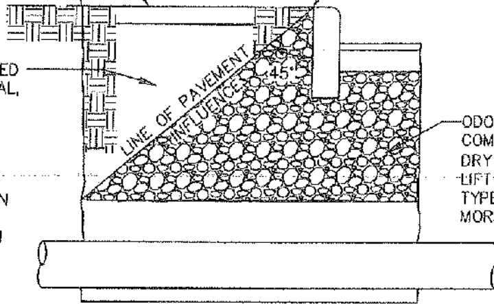
TRENCH DETAIL N.T.S.
